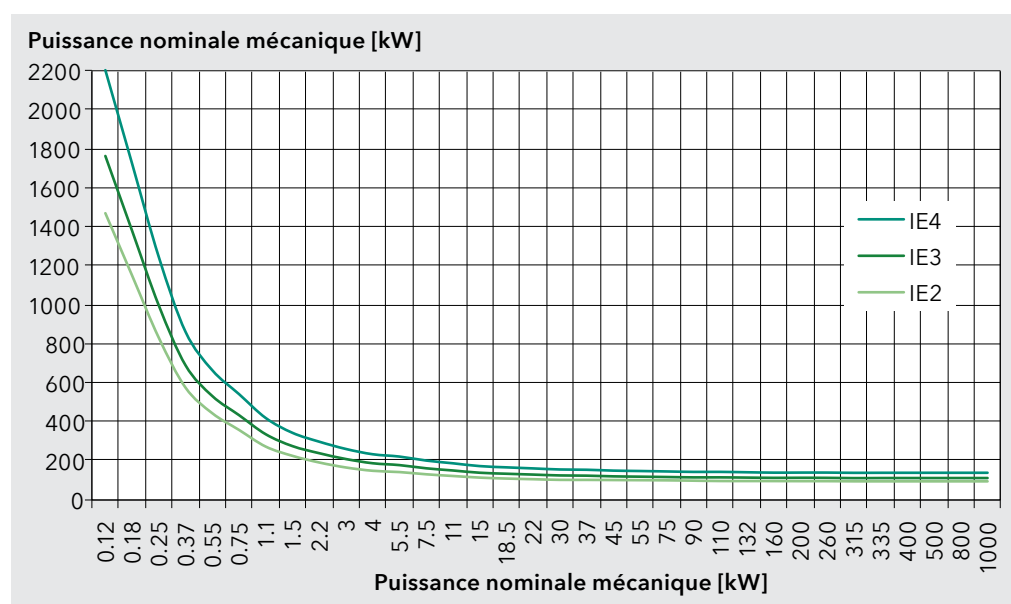
Illustration 1: Prix spécifiques des moteurs en fonction de la puissance nominale pour les trois classes de rendement IE2, IE3 et IE4, 2014. Les indications relatives aux prix des CF figurent dans la fiche technique 11.
